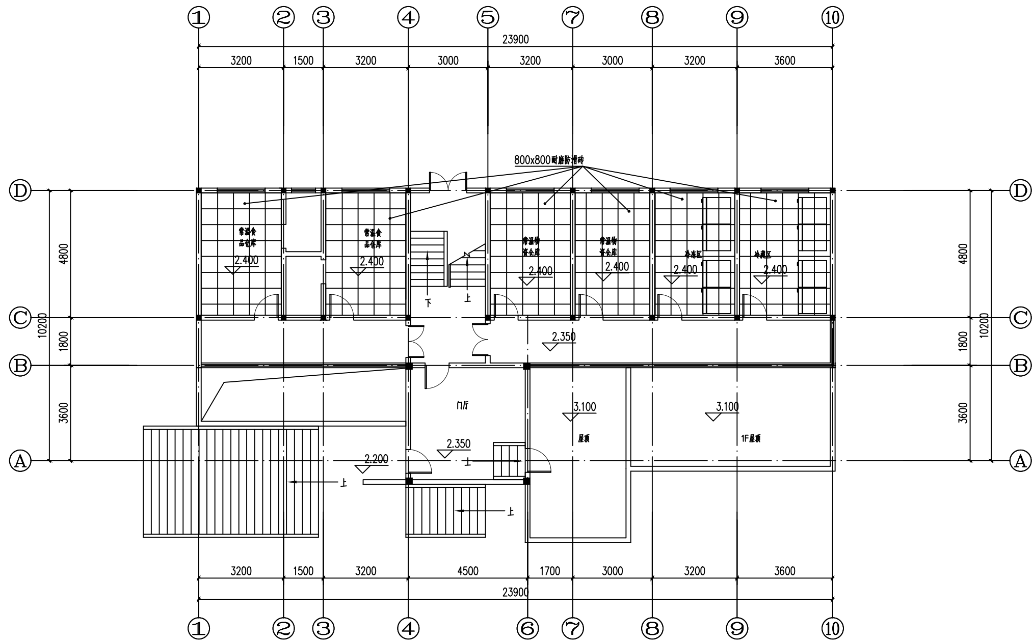
6#楼二平面图 1:100
